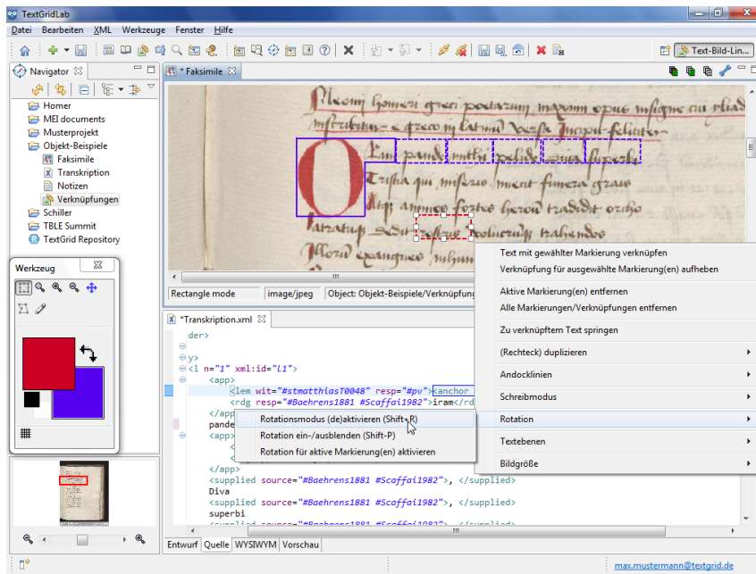
Abbildung 3: Manuellen Rotationsmodus im Kontextmenü aktivieren
