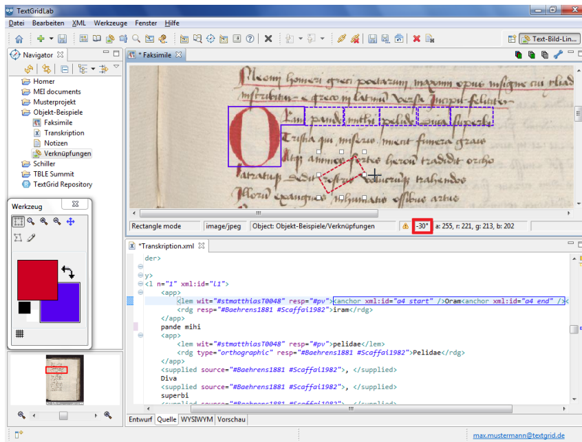
Abbildung 7: Rotationswinkel in der Statusleiste der Bild-Sicht
