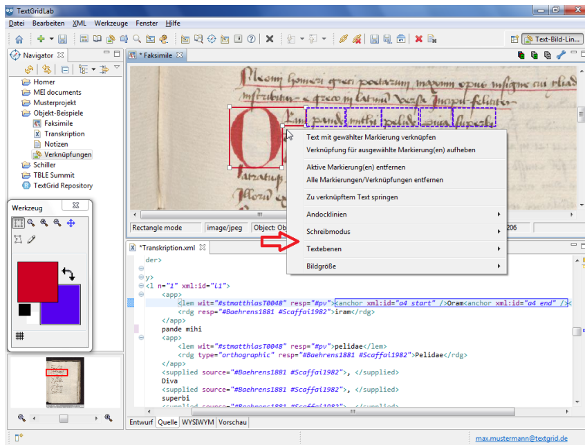
Abbildung 1: Für Polygone kein Rotationsmodus im Menü verfügbar
