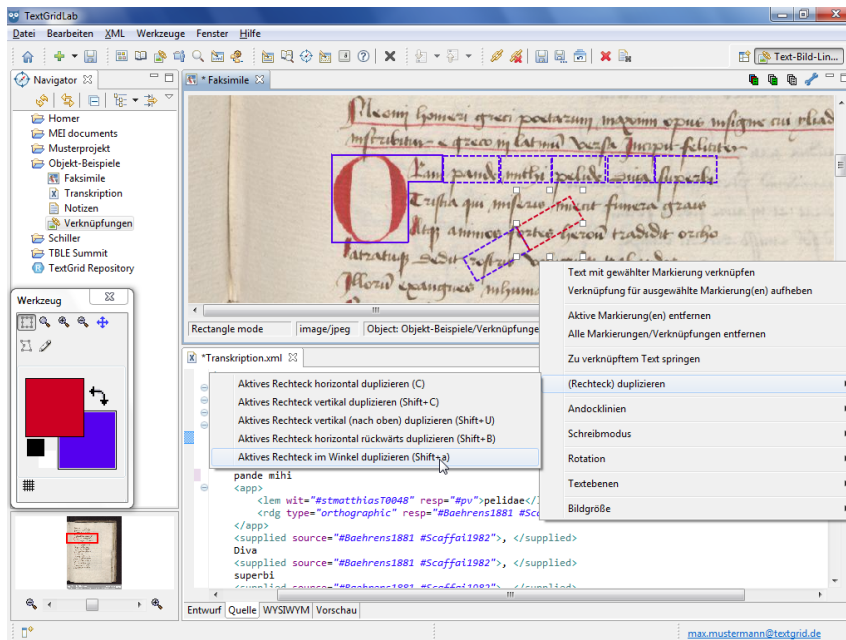
Abbildung 8: Rotierte Markierung im Winkel duplizieren
