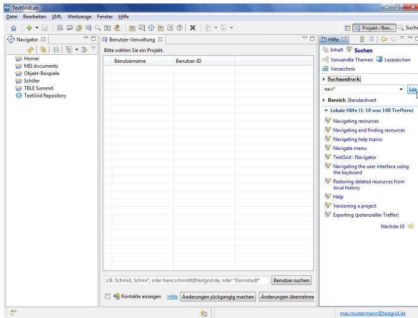
Abbildung 9: Schlüsselwort-Suche
